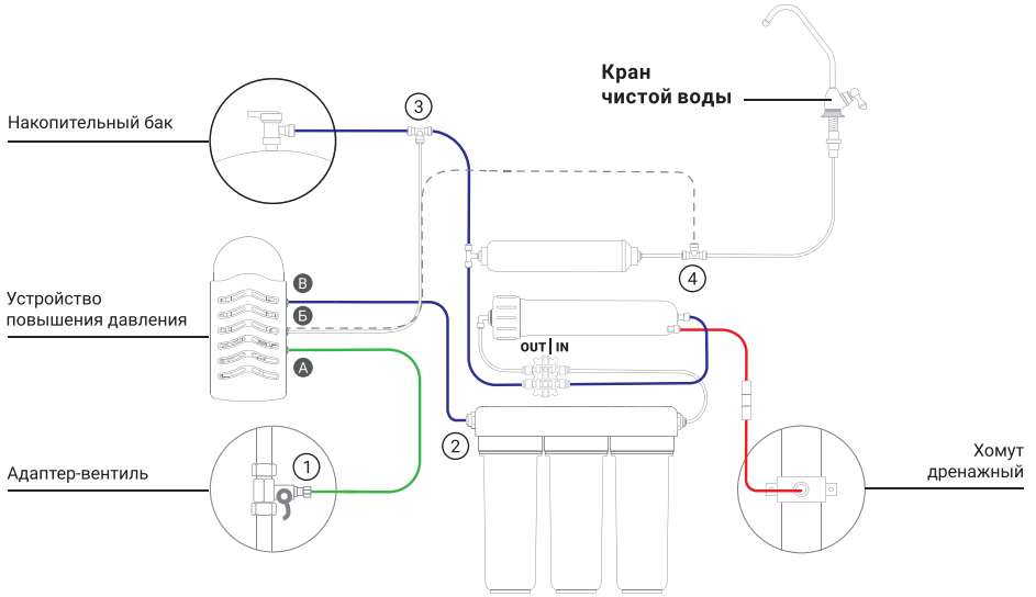
Рис. 5. Схема подключения для систем обратного осмоса Гейзер Престиж, Гейзер Аллегро, Гейзер Нанотек.
