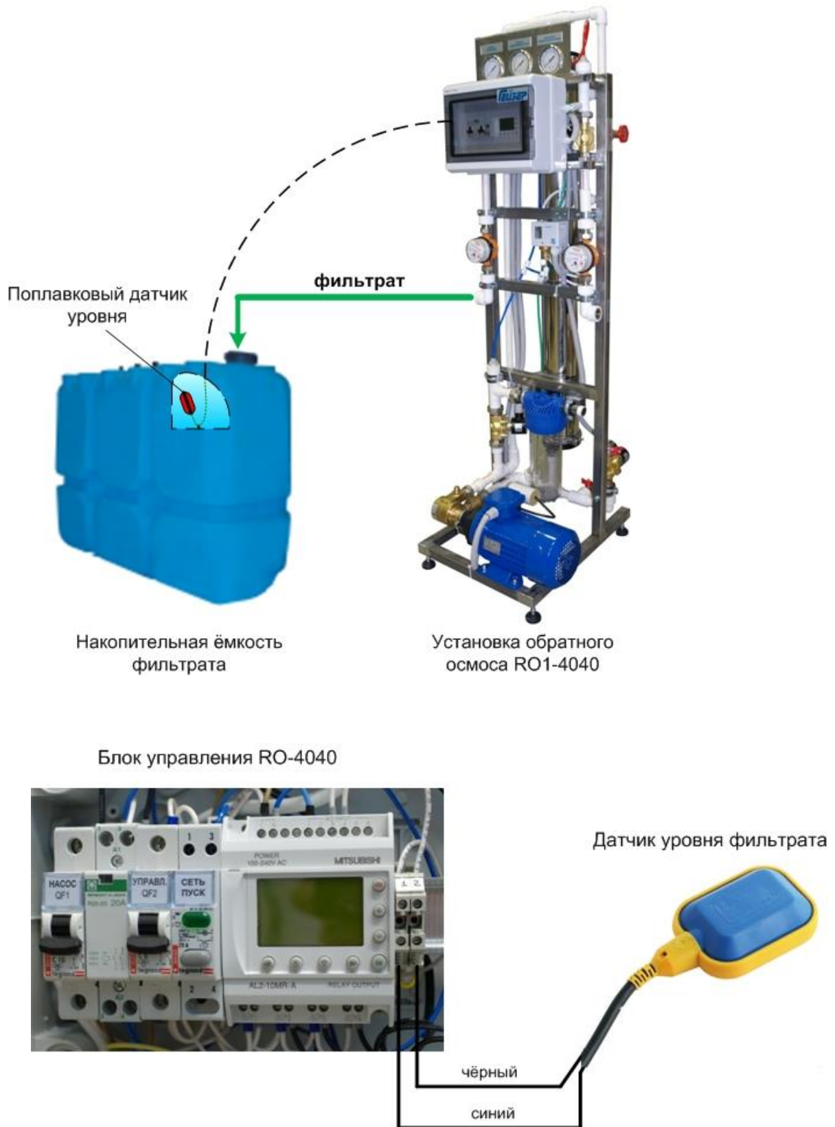
Рис. 5 Подключение одного датчика уровня к установке.
